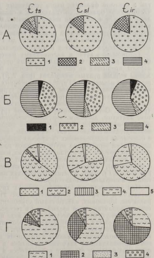
Рис. 2. Соотношение минералов крупноалевритовой фракции (0,1—0,05 мм) алевролитов тискреской (Ets), соэлаской (Esl) и ирбенской (Eir) свит Западной Эстонии. А — минеральный состав легкой фракции: 1 — кварц, 2 — полевые шпаты, 3 — слюды, 4 — аутигенные минералы; Б — основные группы минералов тяжелой фракции: 1 — черные рудные, 2 — прозрачные аллотигенные, 3 — слюды, 4 — аутигенные минералы; В — минеральный состав группы прозрачных аллотигенных тяжелых минералов: 1 — циркон, 2 — турмалин, 3 — гранат, 4 — Ti-минералы, 5 — остальные; Г — минеральный состав группы аутигенных тяжелых минералов: 1 — Ti-минералы, 2 — пирит, 3 — гидроокислы железа, 4 — карбонаты.
