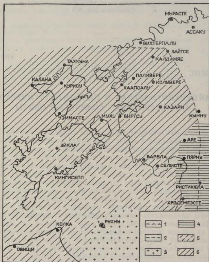
Рис. 1. Нижняя поверхность созлаской свиты с расположением изученных буровых скважин. 1 — северная граница современного распространения отложений созлаской свиты, 2 — предполагаемая восточная граница созлаской свиты, 3 — кристаллический фундамент, 4 — балтийская серия, 5 — люкатская свита, 6 — тискреская свита.
