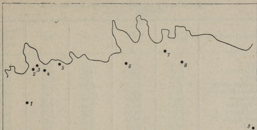
Рис. 1. Местоположение изученных образцов болотных руд. 1 — Раудалу, 2 — Клоостриметса, 3 — Пярнамяэ, 4 — Маарду-Крооднору, 5 — Иыэляхтме-Маннива, 6 — Кахала-Уури, 7 — Тыгу-Рауасоо, 8 — Вийтна-Рауасоо, 9 — Тудусилла.
