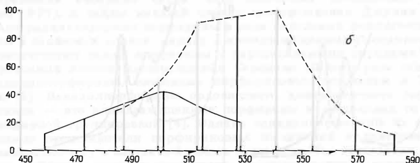
Рис. 2 Интенсивности пиков молекулярных ионов свободных порфириновых оснований (а) и ванадилпорфиринов (б) диктионемового сланца, никелевых порфиринов (в) кукурсита и продуктов их демеаллирования (г)
