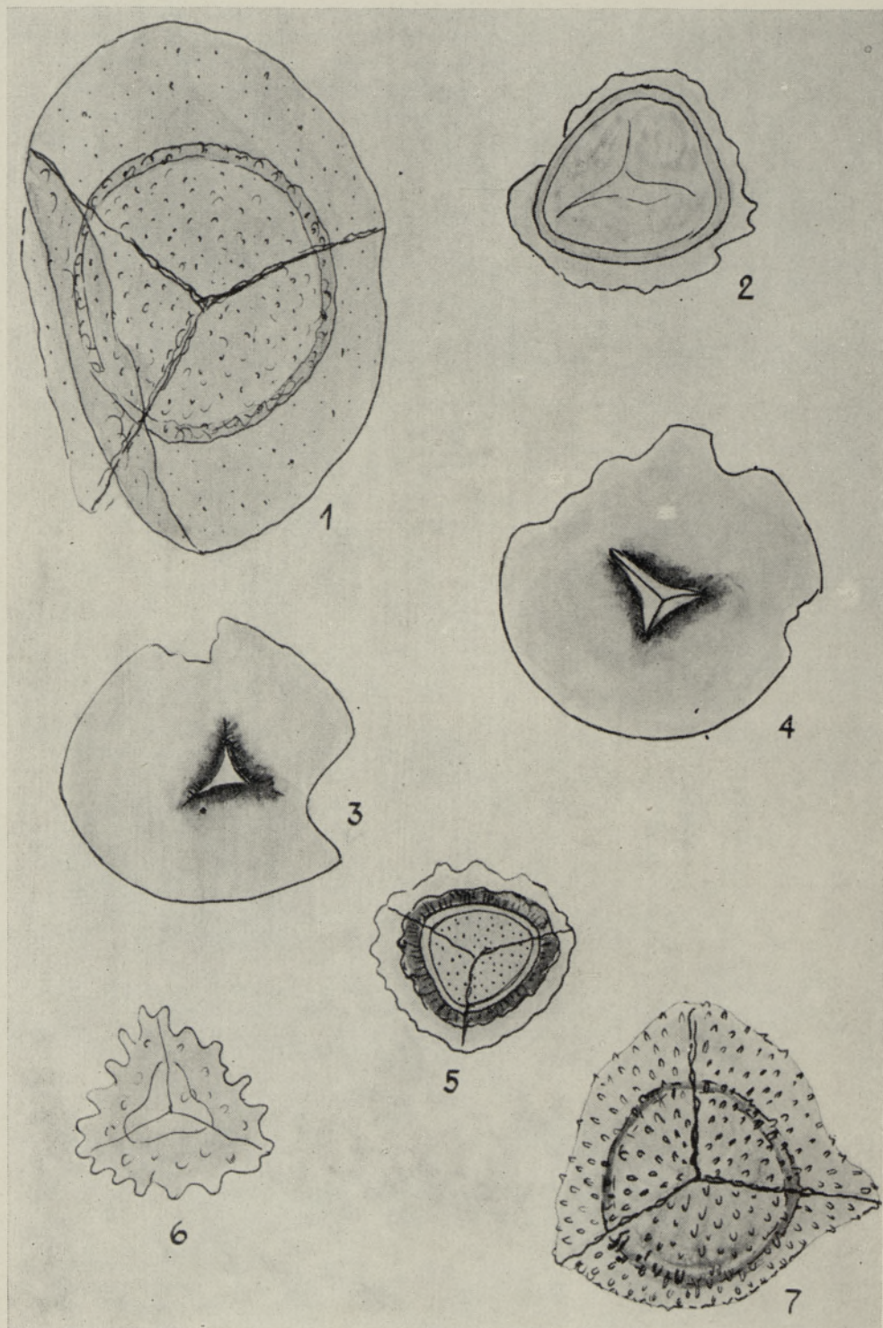
Рис. 2. Переотложенные споры Humenozotriletes sp. sp. (1, 2, 5, 7), Leiotriletes sp., (3, 4) и Acantotriletes sp. (6) в морене на выходах девонских пород южнее оз. Онтарио в Канаде.
