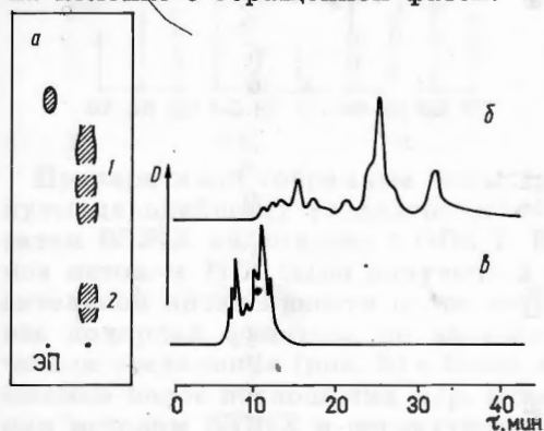
Рис. 3 Хроматограмма ТСХ концентрата ванадилпорфиринов (а): 1 и 2 — зоны (фракции) 1 и 2, ЭП — ванадиловый комплекс этиопорфирина; хроматограммы ВЭЖХ фракций ТСХ 1 (б) и 2 (в)
