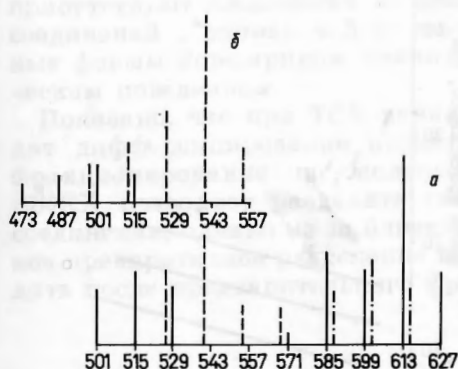
Рис. 4 Масс-спектры фракций ТСХ: a — фракция 1, б — фракция 2. Условные обозначения: сплошная линия — ряд М, пунктирная линия — ряд М-2, точки и тире — ряд М+2
