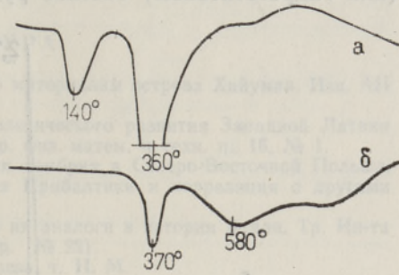
Рис. 1. Термограммы образцов бурой оолитовой железной руды. а — скв. Дурбе-35, гл. 1277 м; б — скв. Павилоста-51, гл. 1365—1369 м.
