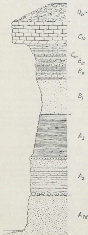
Рис. 9. Разрез кембрийских и нижнеордовикских отложений на мысе Пакерорт. Объяснения см. в тексте.
