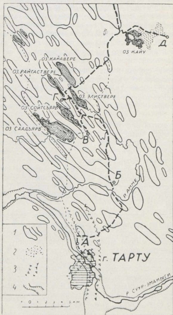
Рис. 2. Схема окрестностей Тарту—Саадъярв. 1 — друмлины; 2 — камни; 3 — погребенные до- лины; 4 — долина р. Суур-Эмайыги. А — пеще- ры Арукюла; Б — карьер Кобрату; В и Г — друмлины у оз. Соитсъярв и оз. Райгаствере; Д— камь у оз. Кайу.
