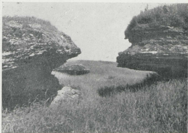
Фиг. 2. Карстовые формы в Костивере.
