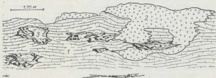
Рис. 10. Разрез биогерма в одном из старых карьеров вблизи ст. Вазалемма.
