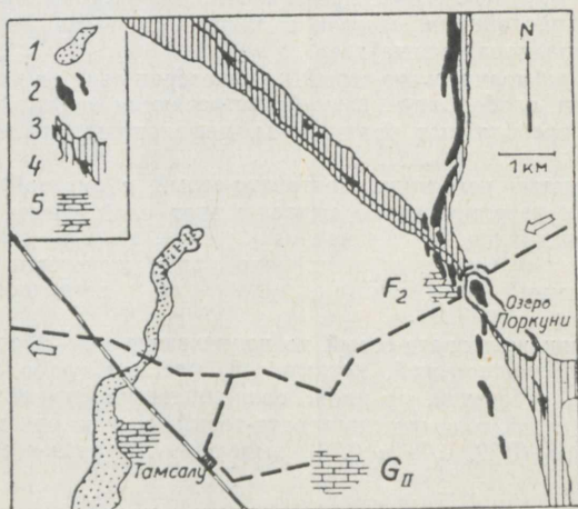
Рис. 7. Схема окрестности Поркуни—Тамсалу. 1 — конечная морена; 2 — озы; 3 — древние долины Поркуни-Нээрути; 4 — направление течения талых вод ледника; 5 — выходы коренных пород поркуниского ( F_2 ) и тамсалуского ( G_{II} ) горизонтов; прерывистой линией показан маршрут экскурсии.
