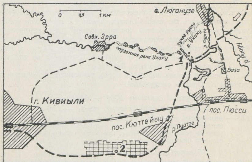
Рис. 4. Схема окрестностей Пюсси—Кивийли. 1 — карстовые родники у Кыргекалас («Высокий берег»); обнажается ухакусский горизонт; 2 — карьер «Кюттейюд»; обнажается кукурзуский горизонт.
