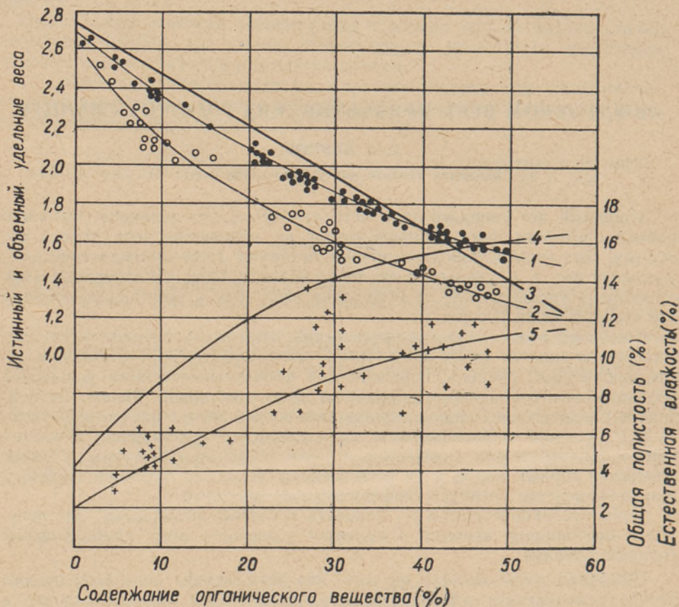
Фиг. 1. Изменение истинного удельного веса, объемного веса, общей пористости и естественной влажности прибалтийских горючих сланцев и переслаивающихся с ними известняков в зависимости от содержания в них органического вещества (точки на графике нанесены по данным таблиц 1 и 3). 1 — истинный удельный вес сухой массы породы по экспериментальным данным; 2 — объемный вес сухой массы породы по экспериментальным данным; 3 — истинный удельный вес сухой массы породы, вычисленный по формуле ГОСТ 2962-45; 4 — общая пористость породы по расчету (в % на сухую массу); 5 — естественная влажность породы (%).
