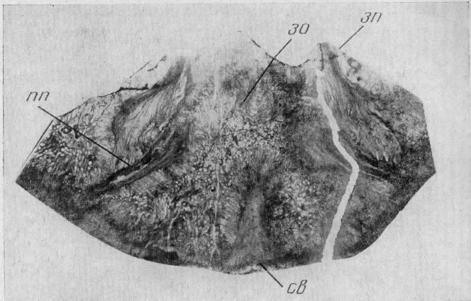
Рис. 2. Bajanhongorella bajanhongorica sp. nov.; экз. № 4534/239, шлиф среза примакущечной части в 2,5 мм от макушки ( \times 15 ); Баянхонгорский выступ, р. Буридуингол, разрез Цагаан-Дэл, слой 2; нижний ашгилл. Обозначения: пп — приямочные пластины, зо — замочный отросток, св — септальный валик, зп — зубные пластины
