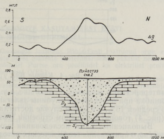
Рис. 3. Аномалия силы тяжести над погребенной долиной у д. Карукиюла (Юго-Западная Эстония) и геологический разрез по данным гравиразведки.
