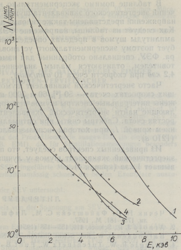
Рис. 3. Интегральные спектры амплитуды собственных шумов некоторых ФЭУ: 1 — ФЭУ-1С № 5901; 2 — ФЭУ-11 № 8301; 3 — ФЭУ-1С № 5798; 4 — ЕМІ 6097 № 16612.
