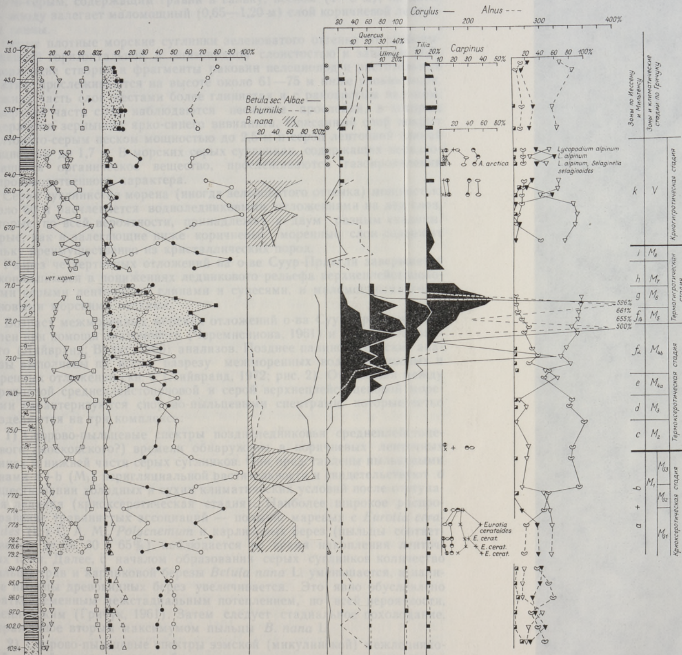
Рис. 2. Спорово-пыльцевая диаграмма плейстоценовых отложений скв. 6 разреза Суур-Прангли. Усл. обозн. см. рис. 1.
