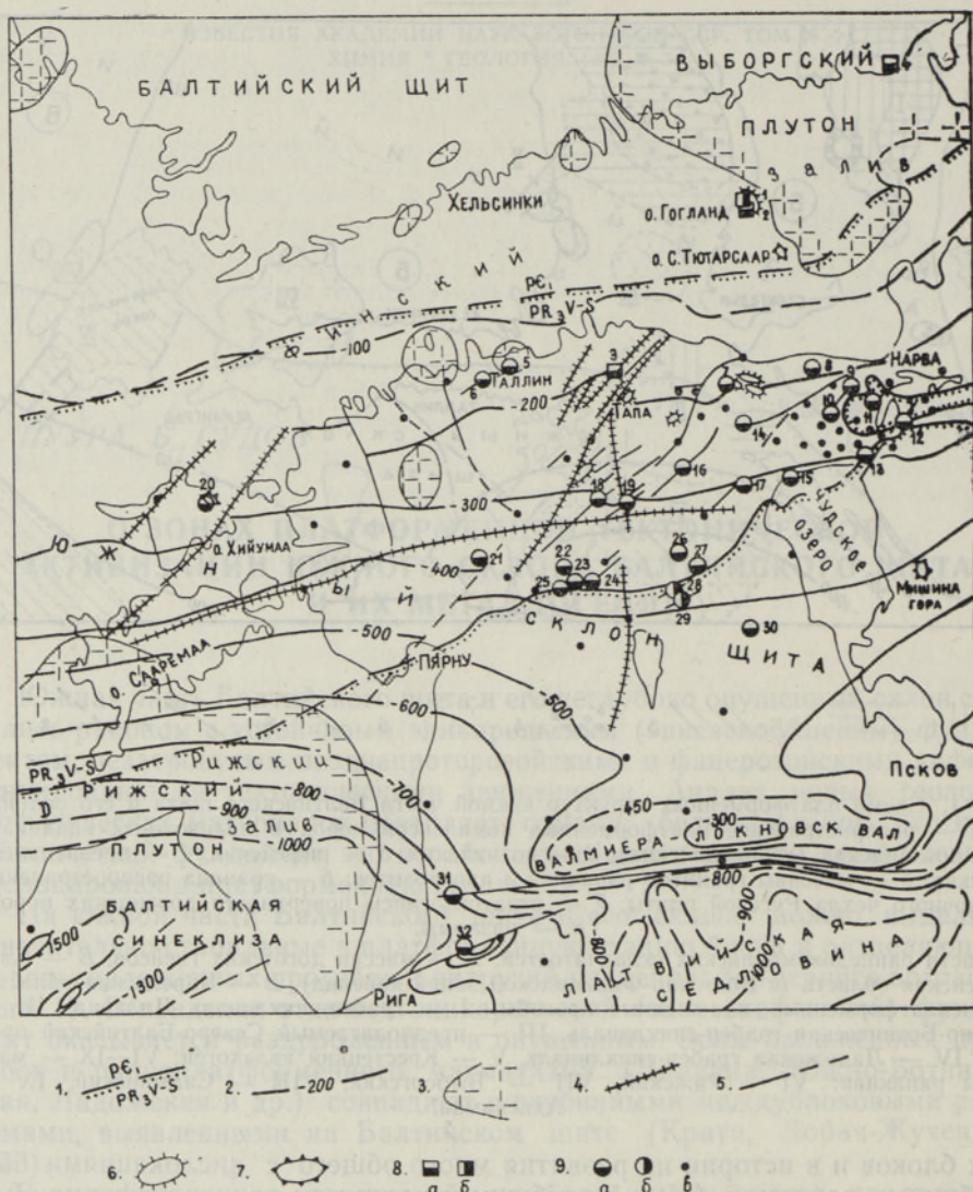
Рис. 2. Схема платформенных дислокаций и проявлений рудной минерализации на южном склоне Балтийского щита: 1 — границы структурных этажей (индексами показан стратиграфический объем); 2 — изгибсы поверхности кристаллического фундамента; 3 — массивы гранитов рапакиви в кристаллическом фундаменте; 4—7 — дислокации: 4 — разрывные нарушения древнего заложения в кристаллическом фундаменте, частично отражающиеся в осадочном чехле, 5 — платформенные разрывные нарушения в кристаллическом фундаменте и осадочном чехле, 6 — локальные поднятия кристаллического фундамента, 7 — кольцевые структуры; 8 — гидротермальные проявления рудной минерализации в кристаллическом фундаменте: а) — полиметаллические, б) — меднополиметаллические; 9 — телотермальные проявления рудной минерализации в кристаллическом фундаменте и осадочном чехле: а) — полиметаллические, б) — меднополиметаллические, в) — находки рудных минералов.
