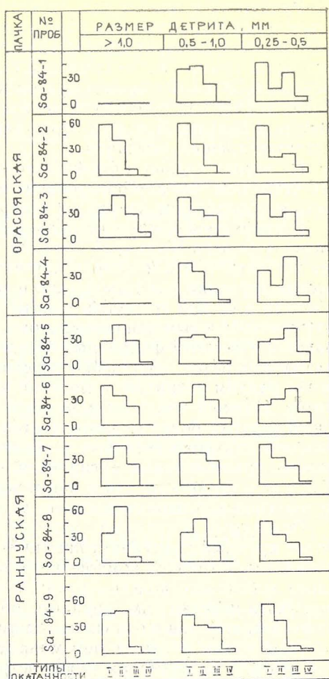
Рис. 2. Распределение типов детрита брахиопод по окатанности в отложениях каллавереской свиты разреза Сака II. Типы окатанности: I — неокатанный, II — слабо окатанный, III — окатанный, IV — хорошо окатанный.
