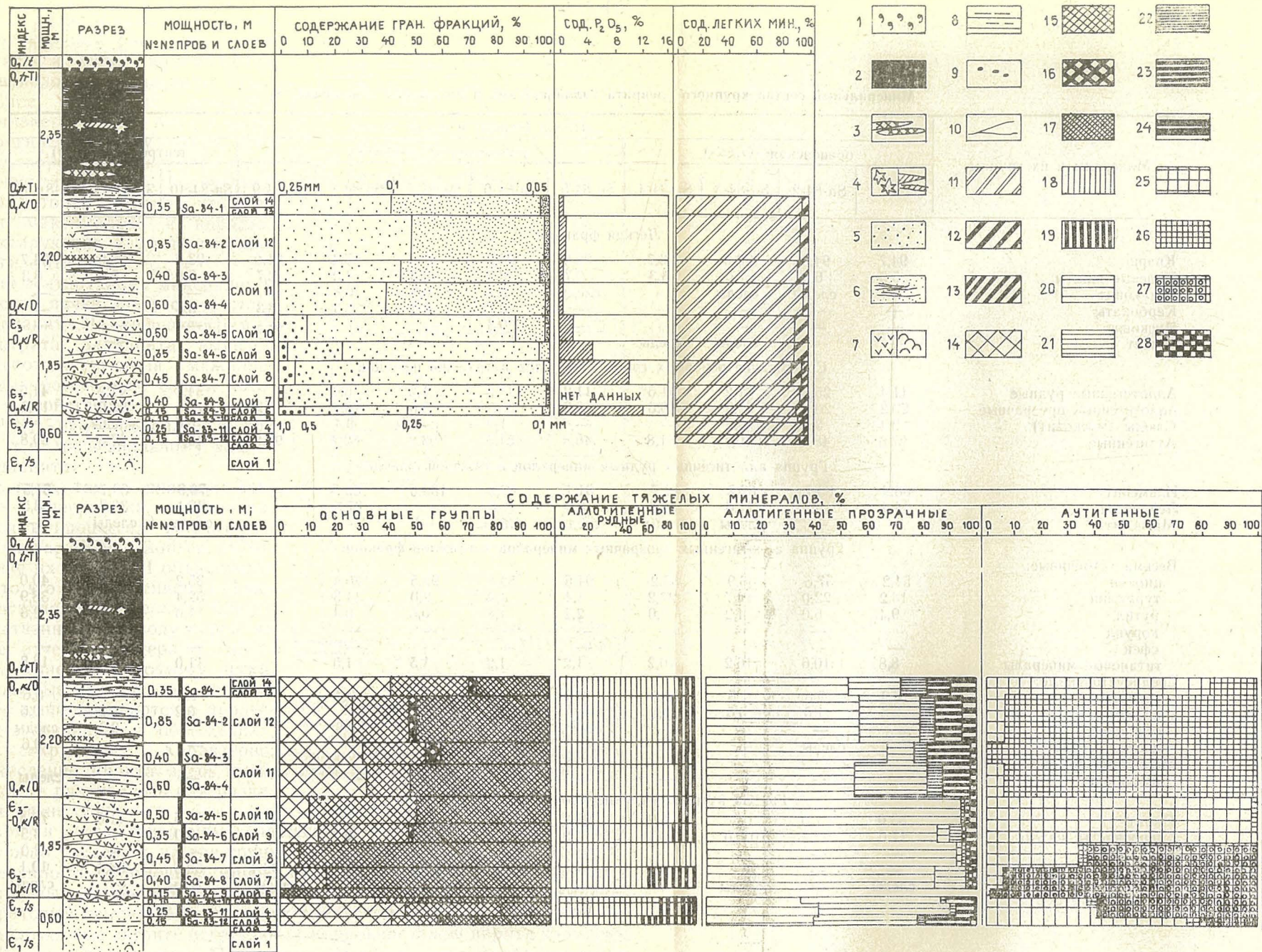
Рис. 1. Литологическая и минералогическая характеристика пограничных кембро-ордовикских отложений разреза обнажения Сака II. 1 — глауконитовый песчаник, 2 — граптолитовый аргиллит, 3 — пиритизированные линзы алевролита, 4 — конкреции антраконита и линзы мучнистого кремнистого материала, 5 — кварцевый песчаник, 6 — алевролит с прослоями граптолитовых аргиллитов, 7 — брахиоподовый детрит и почти целые створки, 8 — прослой глины, 9 — фосфатизированные гальки, 10 — косяя слоистость, 11 — кварц, 12 — полевые шпаты, 13 — карбонаты, 14 — аллотигенные рудные минералы, 15 — аллотигенные прозрачные минералы, 16 — слюды, 17 — аутигенные минералы, 18 — ильменит, 19 — лейкоксен, 20 — циркон, 21 — турмалин, 22 — рутил, 23 — титановые минералы, 24 — остальные минералы (гранаты, апатит, ставролит, дистен), 25 — пирит, 26 — гидроокислы железа, 27 — карбонаты (тяжелой подфракции), 28 — анатаз.
