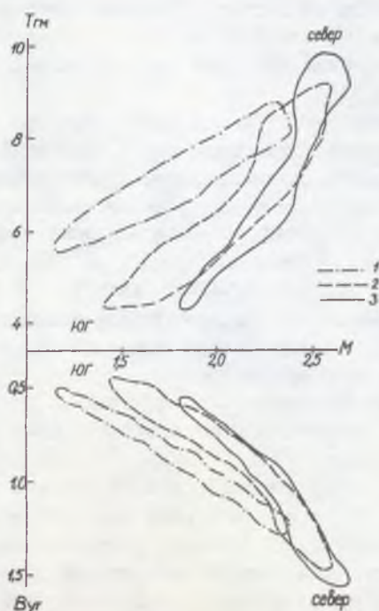
Рис. 5.2.1. Распределение керогенов и битумов в послетремадских ордовикских отложениях Северной и Средней Прибалтики (Пылма, 1983). 1 – кероген кукурсита, 2 – кероген черных аргиллитов, 3 – нефтяные битумы.
