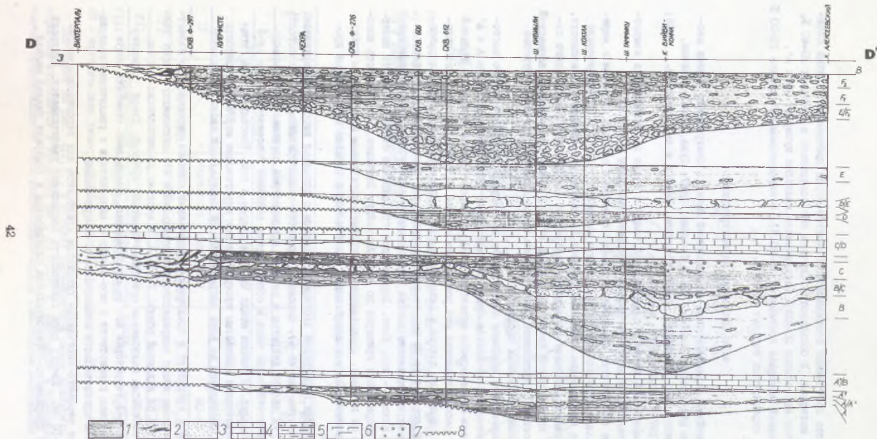
Рис. 4.3.1. Широтный разрез D-D' подразделений промпадки А-Е. 1 - кукурсит, 2 - прерывистые прослои кукурсита, 3 - керогеновый известняк, 4 - глинистый известняк, 5 - сильноглинистый известняк, 6 - мергель, 7 - ходы илоедов, 8 - поверхности перерыва.
