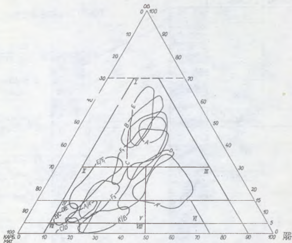
Рис. 4.2.1. Классификация пород промышленной пачки кукурсита А-Р 2 по вещественному составу. Поля I-VIII см. табл. 4.2.т. Контурными линиями показан состав отдельных слоев по данным опробования промпачки в действующих карьерах и шахтах Эстонского и Ленинградского месторождений.
