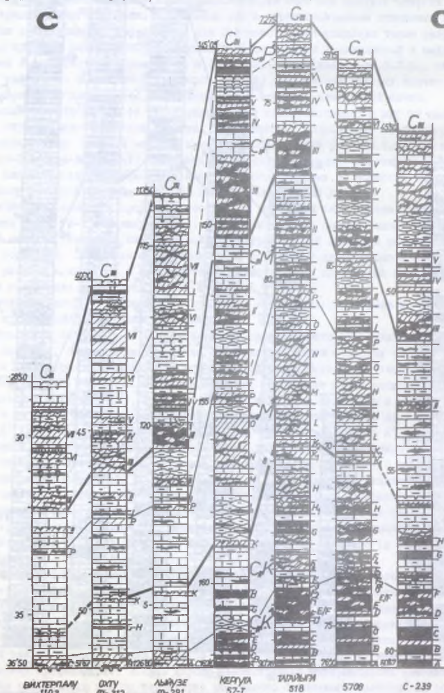
Рис. 3.2.3. Сопоставление разрезов курузеских отложений ( C_{II} ) по широтному профилю С-С'. Усл. обозн. см. рис. 3.1.3.
