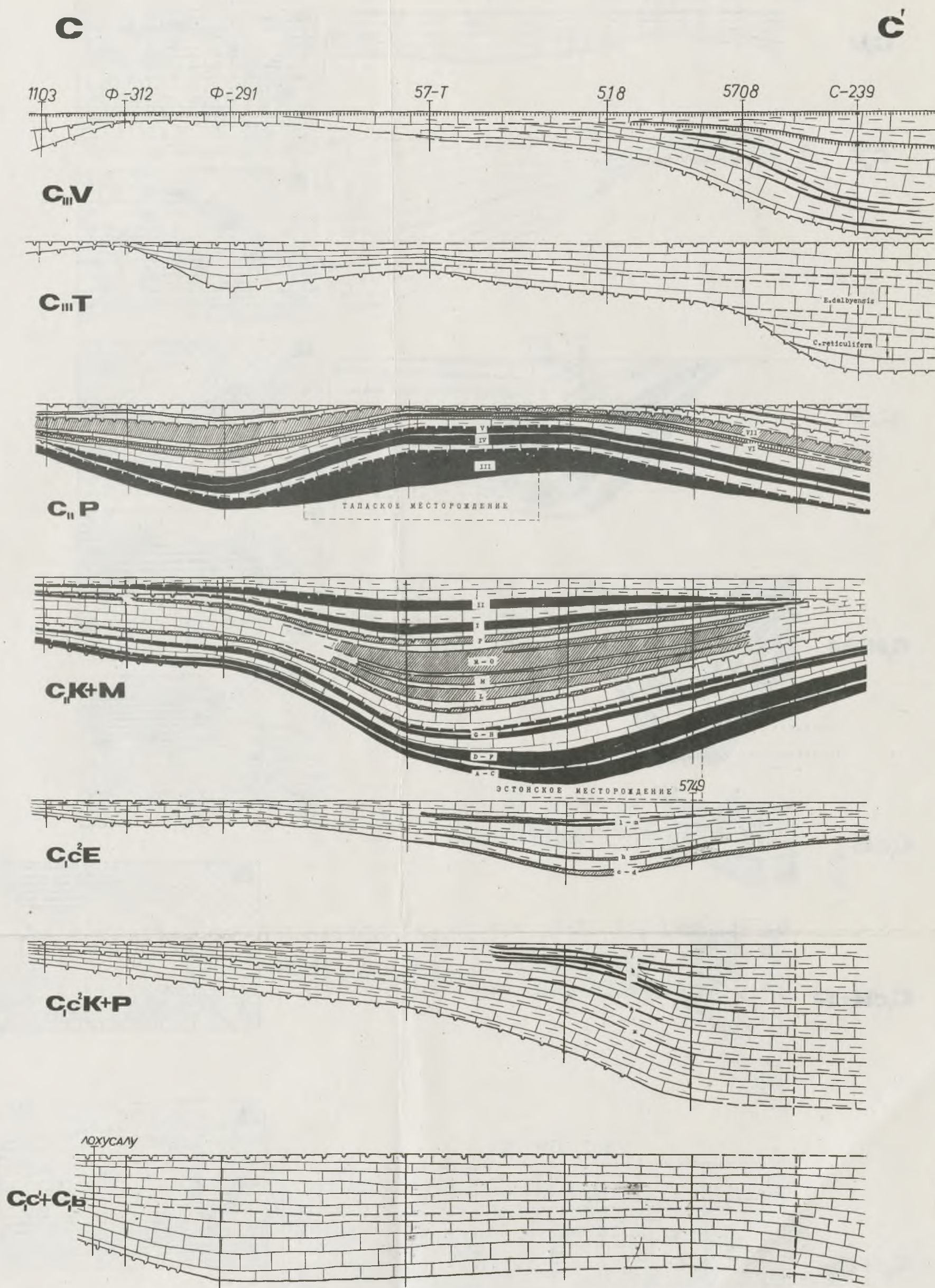
Рис. 5.1.2. Позиция кукуерситовых слоев стратиграфических подразделений C I 1 - C III в широтном профиле C-C'. Усл. обозн. см. рис. 5.1.1.
