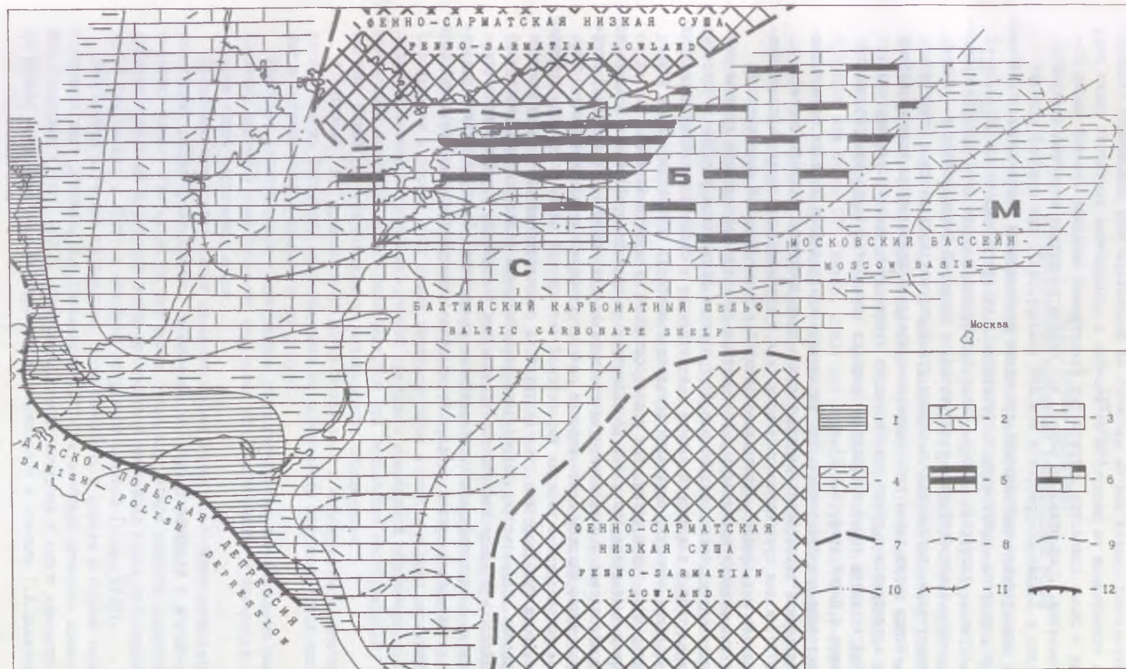
Рис. 5.2.2. Литолого-палеогеографическая схема Балтийского бассейна в главную эпоху кукерситонакопления ( Nemograptus gracilis - время, средний ордовик). 1 - граптолитовые аргиллиты, 2 - глинистые детритистые известняки, 3 - известковые мергели, 4 - детритистые известковые мергели, 5 - богатые проявления кукерсита, 6 - бедные проявления кукерсита, 7 - предполагаемая граница ареала седиментации, 8 - эрозионная граница отложений, 9 - граница зоны максимального кукерситонакопления, 10 - внешняя граница ареала кукерситонакопления, 11 - граница распространения фауны: С - скандинавской, Б - восточно-балтийской, М - московской; 12 - линия Торнквиста (граница платформы).
