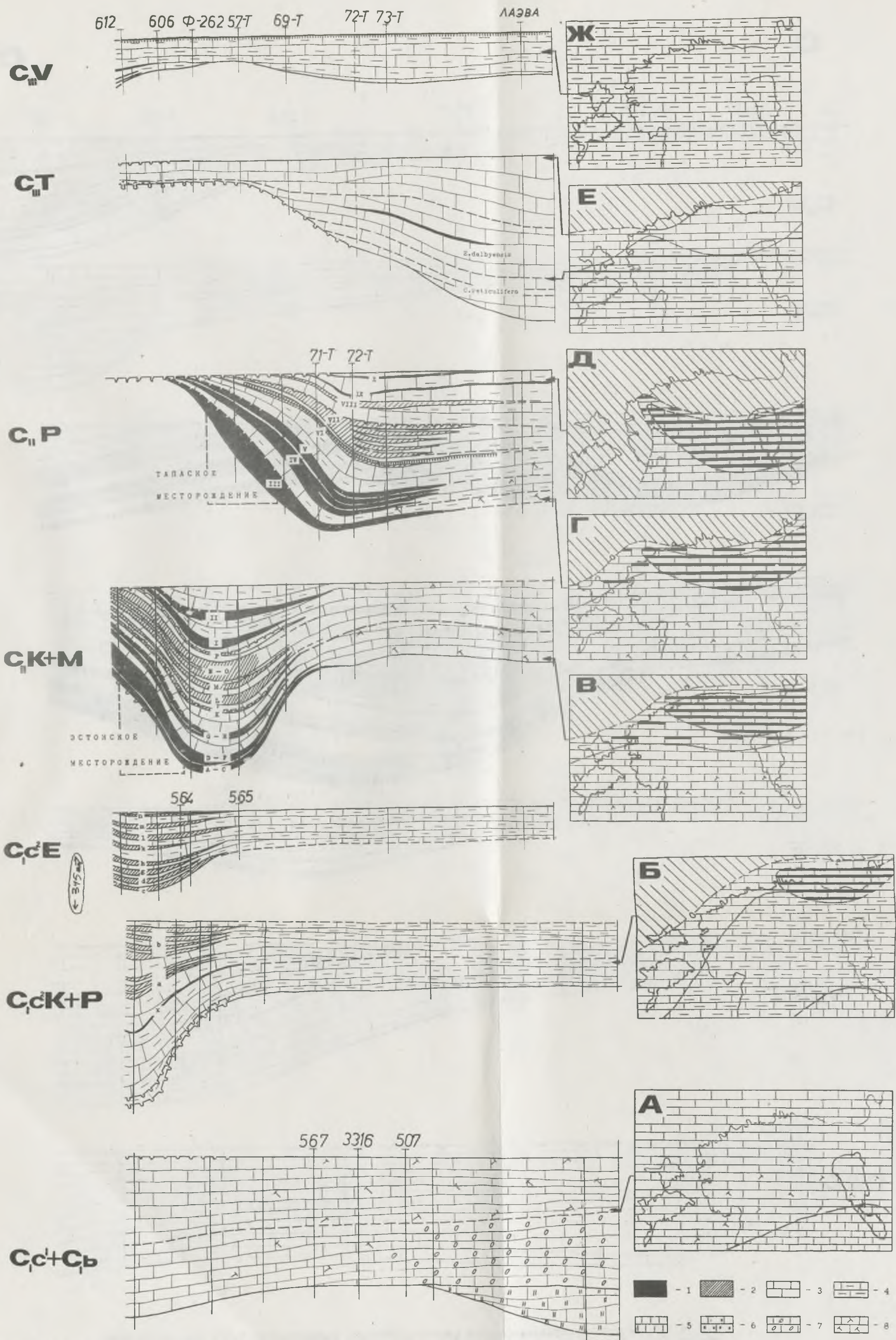
Рис. 5.1.1. Позиция кукурситовых слоев в опорном меридиональном профиле (в полосе вдоль профиля А-А') стратиграфических подразделений C_{II}P - C_{III} (слева) и литологические схемы отдельных моментов истории кукурситонакопления в ранневируское время (справа) I-2 - слои кукурсита относительно богатого (1) и относительно бедного (2) керогеном, 3-8 - известняки: относительно чистые (4), афанитовые (5), пестроцветные (6), с ооидами (7), с пиритизированным детритом (8), 9-10 - распространение кукурсита (9) и керогеновых и керогенистых пород (10), II - отсутствие седиментации (твердое известняковое дно), I2 - слой метабентонита, I3 - поверхность перерыва. Объяснения к литологическим схемам А-Ж см. в тексте.
