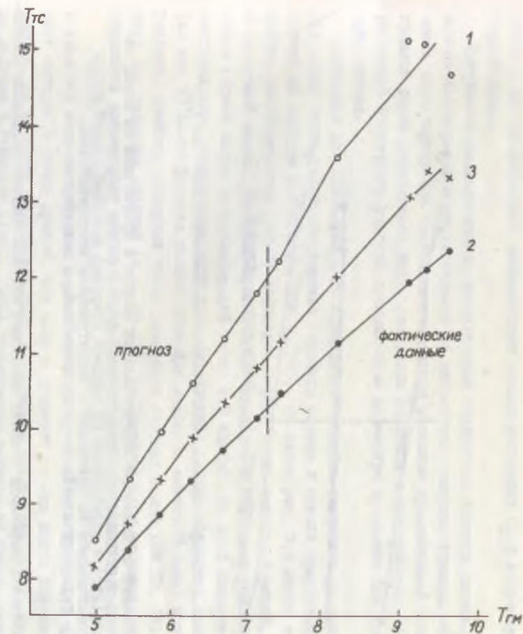
Рис. 7.4. Фактическая по балансам обогатительных фабрик и прогнозная на новых неосвоенных участках месторождений теплота сгорания товарных сортов сланца ( T_{tc} ), МДж/кг в зависимости от теплоты сгорания исходной горной массы промышленной пачки ( T_{gm} ), разрабатываемой на Эстонском и Ленинградском месторождениях, МДж/кг. Сорт сланца: 1 - технологический, 2 - энергетический, 3 - суммарно.
