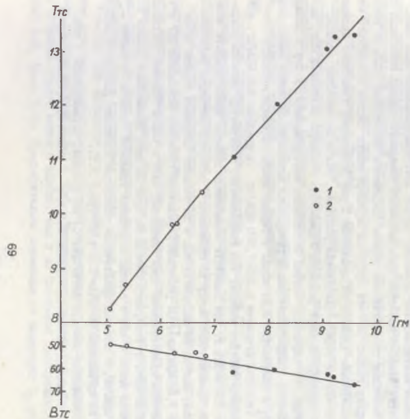
Рис. 7.3. Зависимость теплоты сгорания суммарно энергетического и технологического сортов товарного сланца, МДж/кг ( T_{tc} ) и выхода суммарно этих сортов товарного сланца из горной массы, % ( B_{tc} ) в зависимости от теплоты сгорания исходной горной массы, МДж/кг ( T_{gm} ) по промышленной пачке горючего сланца на Эстонском и Ленинградском месторождениях. 1 - по фактическим данным действующих шахт, 2 - по прогнозу для периферических частей бассейна.
