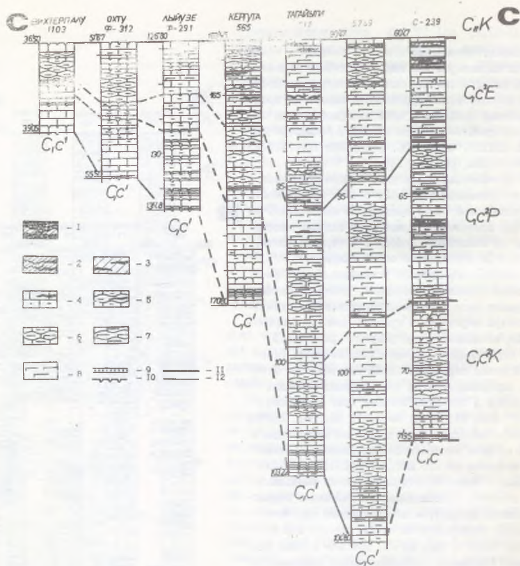
Рис. 3.1.3. Сопоставление разрезов верхнеухакусских отложений ( C_{1c}^2 ) по широтному профилю С-С'. 1 - кукурсит с комками керогенового известняка, 2-6 - известняки; керогеновый и керогенистый с прослоями и линзами кукурсита (2), керогенистый с линзами кукурсита (3), слабоглинистый с линзами кукурсита (4), среднеглинистый комковатый, с линзами кукурсита (5), известняк, сильноглинистый (до известкового мергеля), мелкокомковатый (6), 7 - известковый мергель, мелкокомковатый, 8 - известковый мергель, массивный, 9 - слой метабентонита, 10 - поверхность перерыва, 11 - граница пачек, 12 - граница подпачек.
