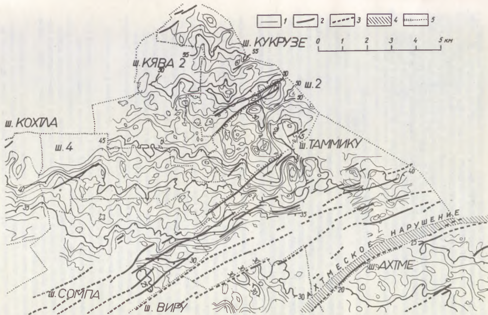
Рис. 6.1.3. Схема структуры сланцевосных отложений по данным маркшейдерских нивелировок. 1 - стратозиогипсы подошвы кукрузе-ского горизонта, 2-3 - закарстованные зоны по данным горных работ (2) и электроразведки (3), 4 - Ахтмеское нарушение, 5 - границы шахт.
