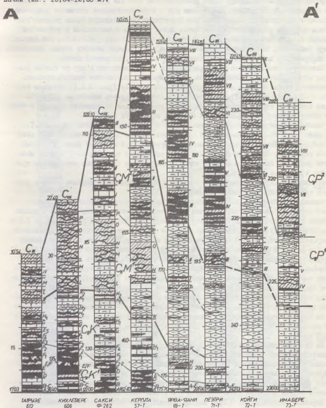
Рис. 3.2.1. Сопоставление разрезов кукурузеских отложений ( C_{II} ) по Тамсалускому меридиональному профилю А-А'. Усл. обозн. см. рис. 3.1.3.
