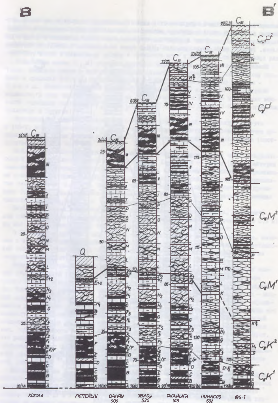
Рис. 3.2.2. Сопоставление разрезов кукурузеских отложений ( C_{II} ) по Кивиньдскому меридиональному профилю В-В'. Усл. обозн. см. рис. 3.1.3.
