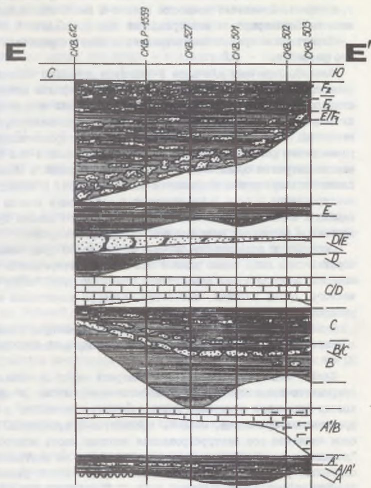
Рис. 4.3.2. Субмеридиональный разрез Е-Е' промпачки А-Р 2 . Усл. обозн. см. рис. 4.3.1.
