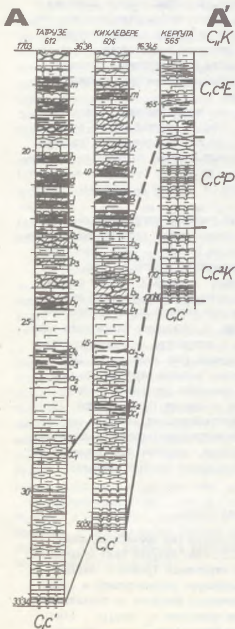
Рис. 3.1.1. Сопоставление разрезов верхнеухакусских отложений ( C_1C_2 ) по Тамсалускому меридиональному профилю А-А'. Усл. обозн. см. рис. 3.1.3. Местоположение профилей см. рис. 1.1.
