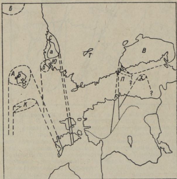
Рис. 3. Распространение руководящих валунов во время невской стадии последнего оледенения. Условные обозначения те же, что на рис. 2.
