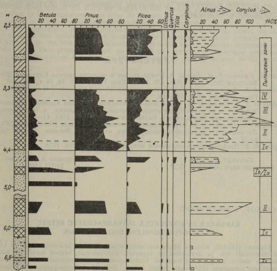
Рис. 3. Нарушение стратификации слоев нижнего интервала перемещенных ливнинских озерных отложений скв. 2 разреза Кырвекюла. (Усл. обозн. см. рис. 1.)
