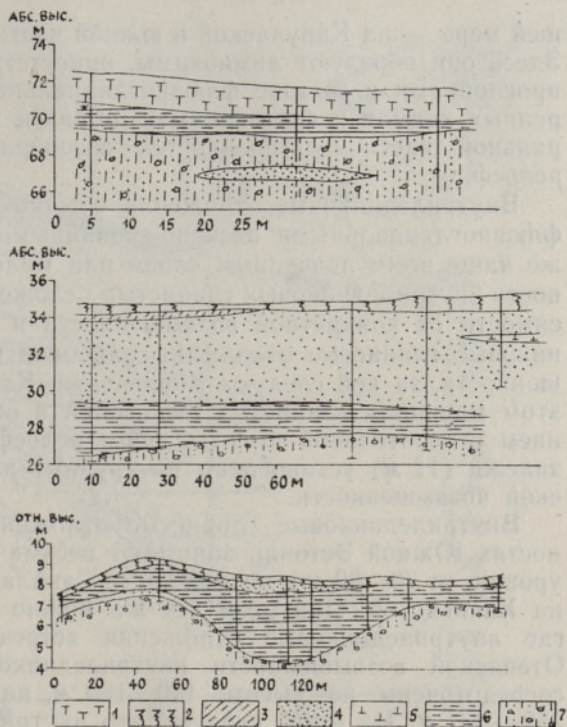
Рис. 2. Условия залегания приледниковых отложений: а — в окрестностях г. Выру; б — во впадине оз. Вуртсъярв; в — в долине р. Тохври (по данным Х. Пальме). 1 — насыль; 2 — почва; 3 — алеврит (голоценовый); 4 — песок; 5 — озерная известь; 6 — ленточная глина; 7 — супесчаная морена.
