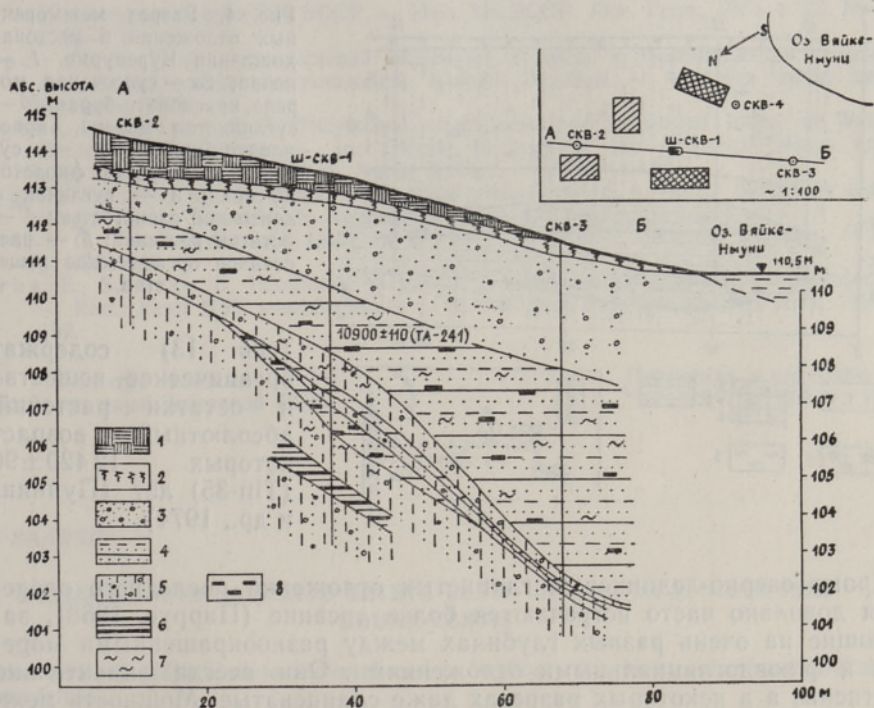
Рис. 3. Разрез межхолмовых отложений в местонахождении Нюуни-Пезду. 1 — насыпь; 2 — почва; 3 — гравий; 4 — переслаивание песчаных и глинистых слоев; 5 — морена; 6 — ленточная глина; 7 — рассеянное органическое вещество; 8 — остатки растений и древесины.
