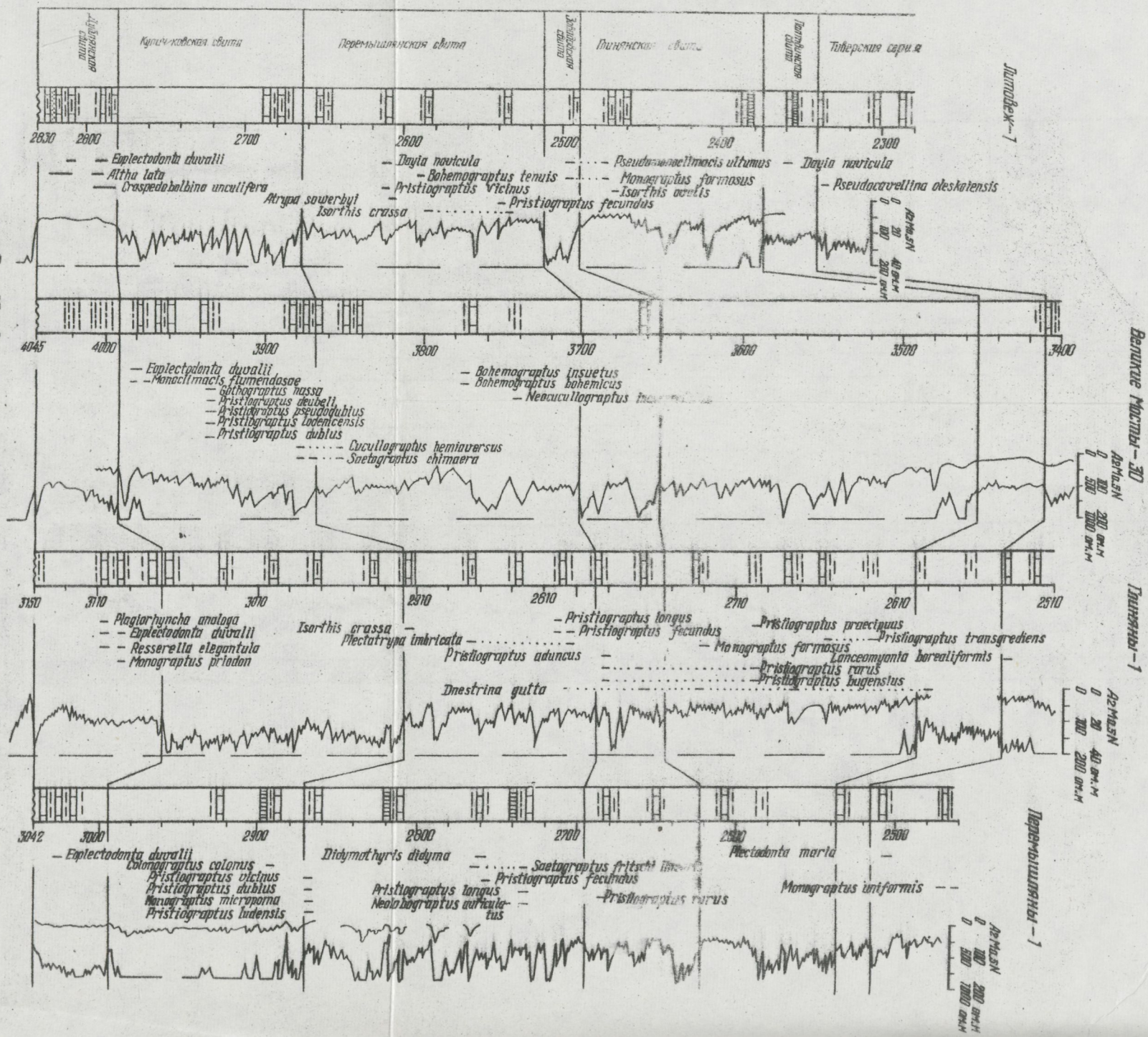
Рис. 25. Сопоставление разрезов скалки по профилю VIII-VII. Условные обозначения см. на рис. 12.
