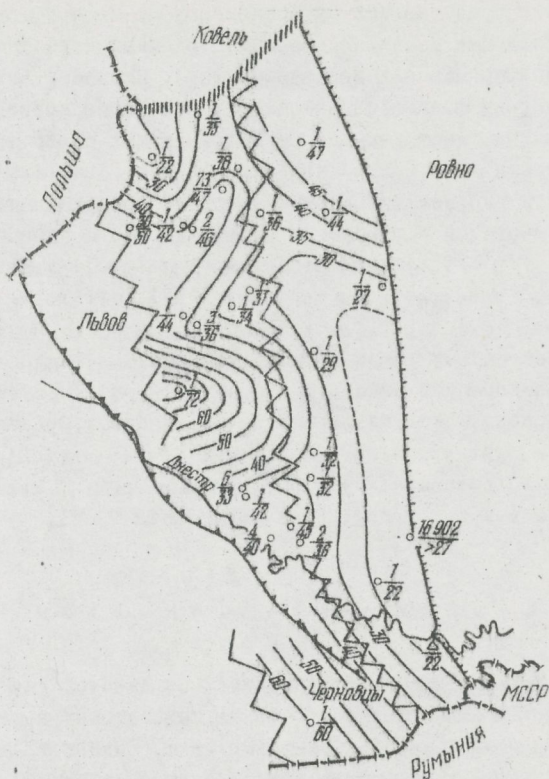
Рис.18. Изопахиты пригородокской и завадовской свит. Условные обозначения см.на рис.13.
