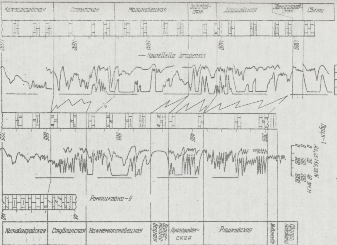
Рис. 20. Сопоставление разрезов скважин по профилю У-У. Условные обозначения см. на рис. 12.
