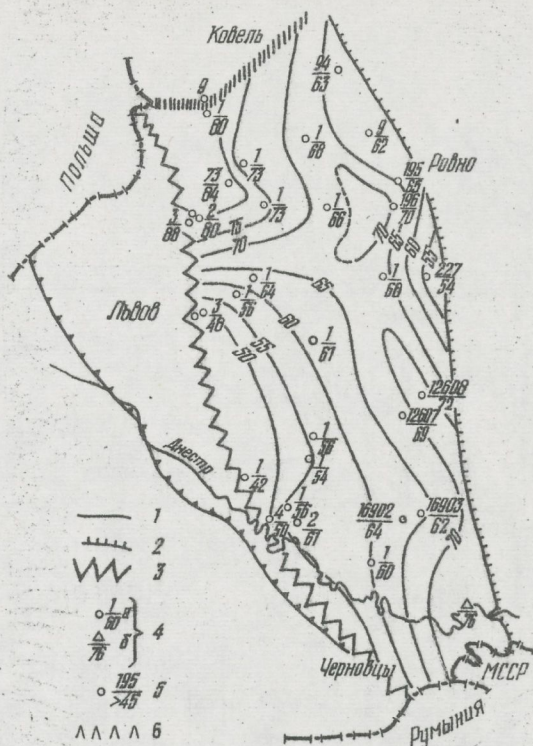
Рис.13. Изопахиты китайгородской свиты:
