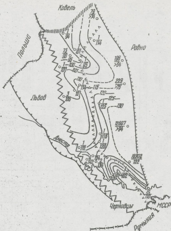
Рис.17. Изопахиты малиновецкой свиты. Условные обозначения см.на рис.13.
