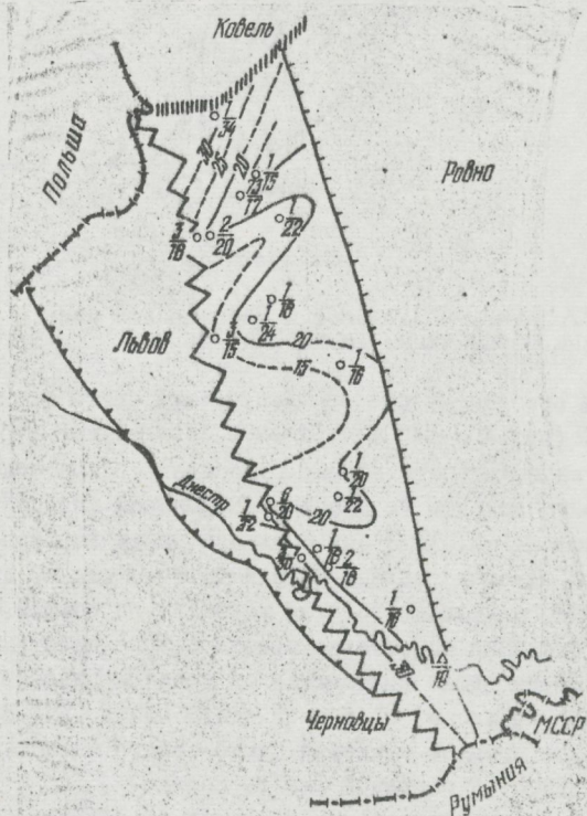
Рис.22. Изопахиты звенигородской свиты. Условные обозначения см. на рис.13.
