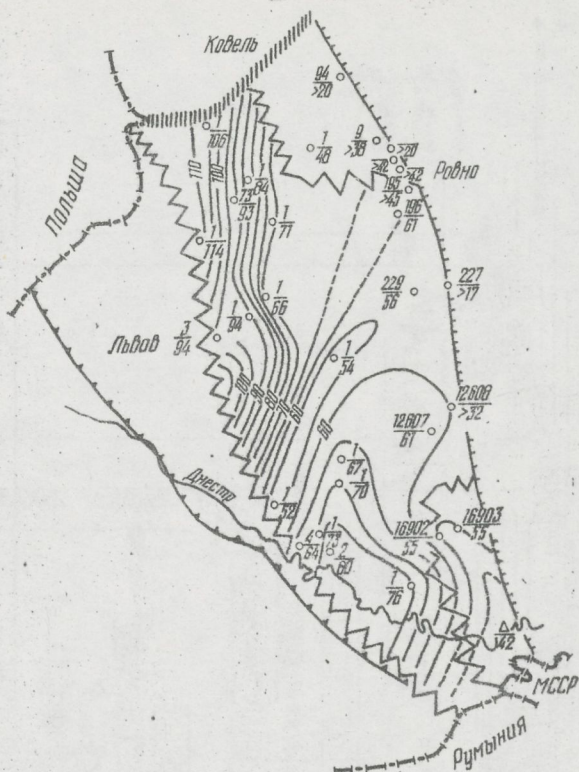
Рис.15. Изопахты баговицкой, стрыпской и стублинской свит. Условные обозначения см. на рис.13.
