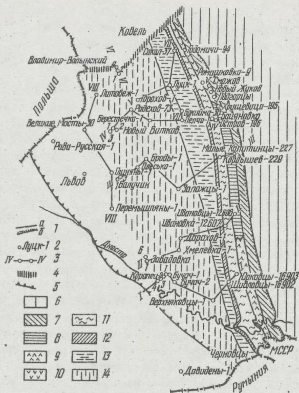
Рис. II. Схематическая геологическая карта додевонской поверхности западного склона Украинского щита и восточного борта Львовского палеозойского прогиба:
