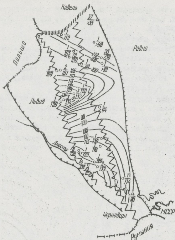
Рис. 21. Изопахиты рашковской и дараховской свит. Условные обозначения см. на рис. 13.
